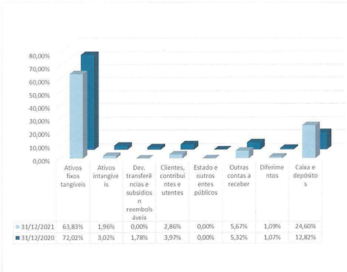
Gráfico 1 - Composição Ativo
